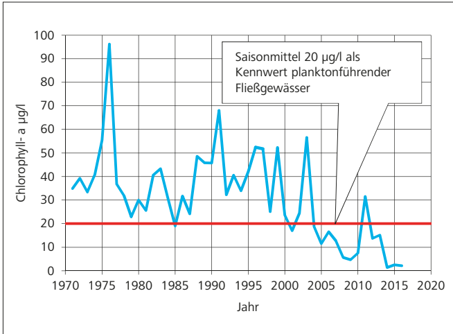
Bild 5.5: Jahresmittelwerte des Chlorophyll-a-Gehalts in der Ruhr bei Essen Rellinghausen in der Vegetationsperiode April bis Oktober der Jahre 1971 bis 2016 Fig. 5.5: Annual means of the chlorophyll a concentration in the Ruhr at Essen-Rellinghausen during vegetation period (April to October), 1971 to 2016
