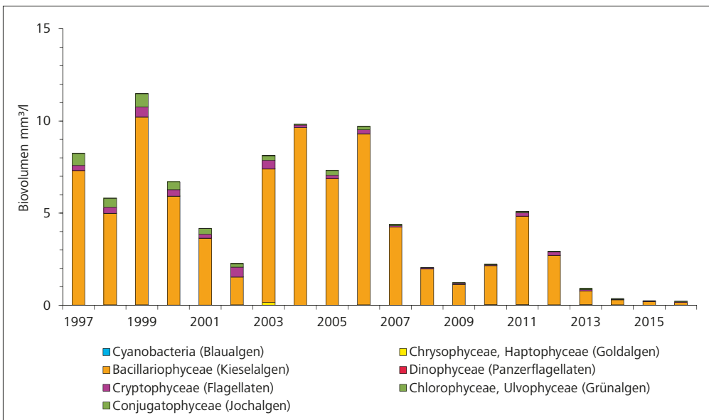
Bild 5.6: Phytoplankton in der Ruhr bei Essen-Rellinghausen (Jahresmittelwerte des Biovolumens der Jahre 1997 bis 2016) Fig. 5.6: Phytoplankton in the Ruhr River at Essen-Rellinghausen (yearly means of biovolume 1997 to 2016)
